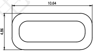
带防水圈示意图
